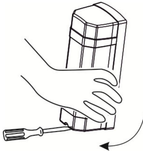
Рисунок 2.8 - Порядок отсоединения крышки от базового основания
