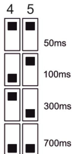
Рисунок 2.12 - Положение переключателей времени прерывания
