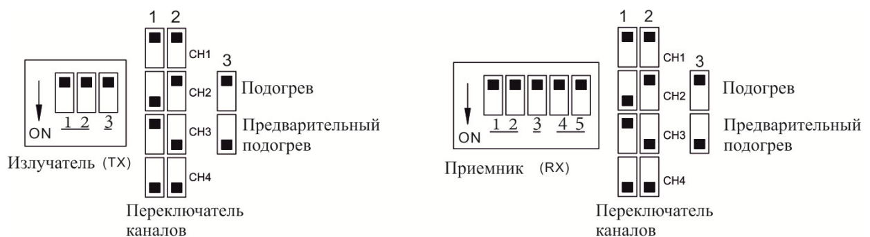
Рисунок 2.11 - Переключатель каналов
